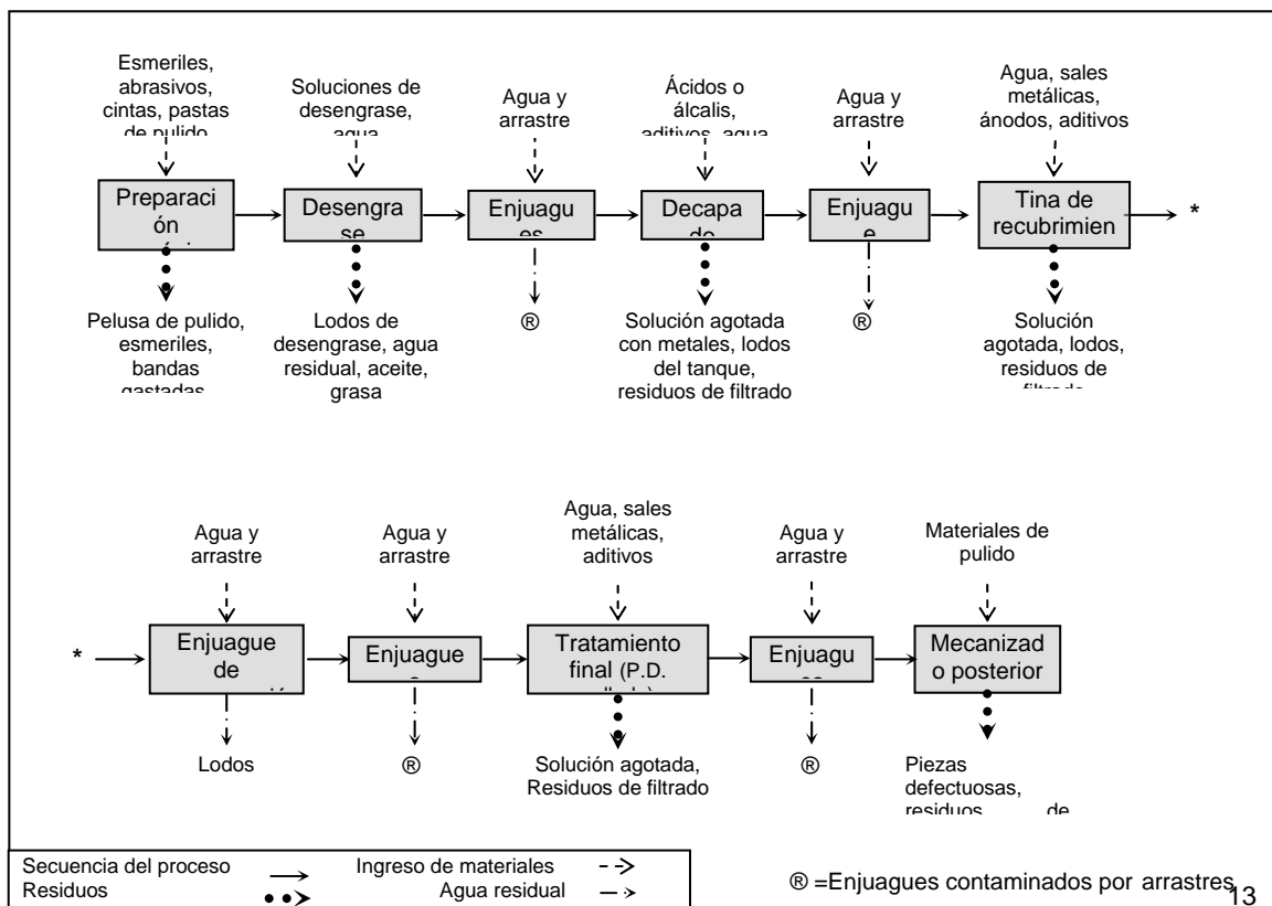
Figura N° 1: Ejemplo de un diagrama de flujo simplificado con diversas operaciones unitarias, del rubro de la Galvanoplastia.
