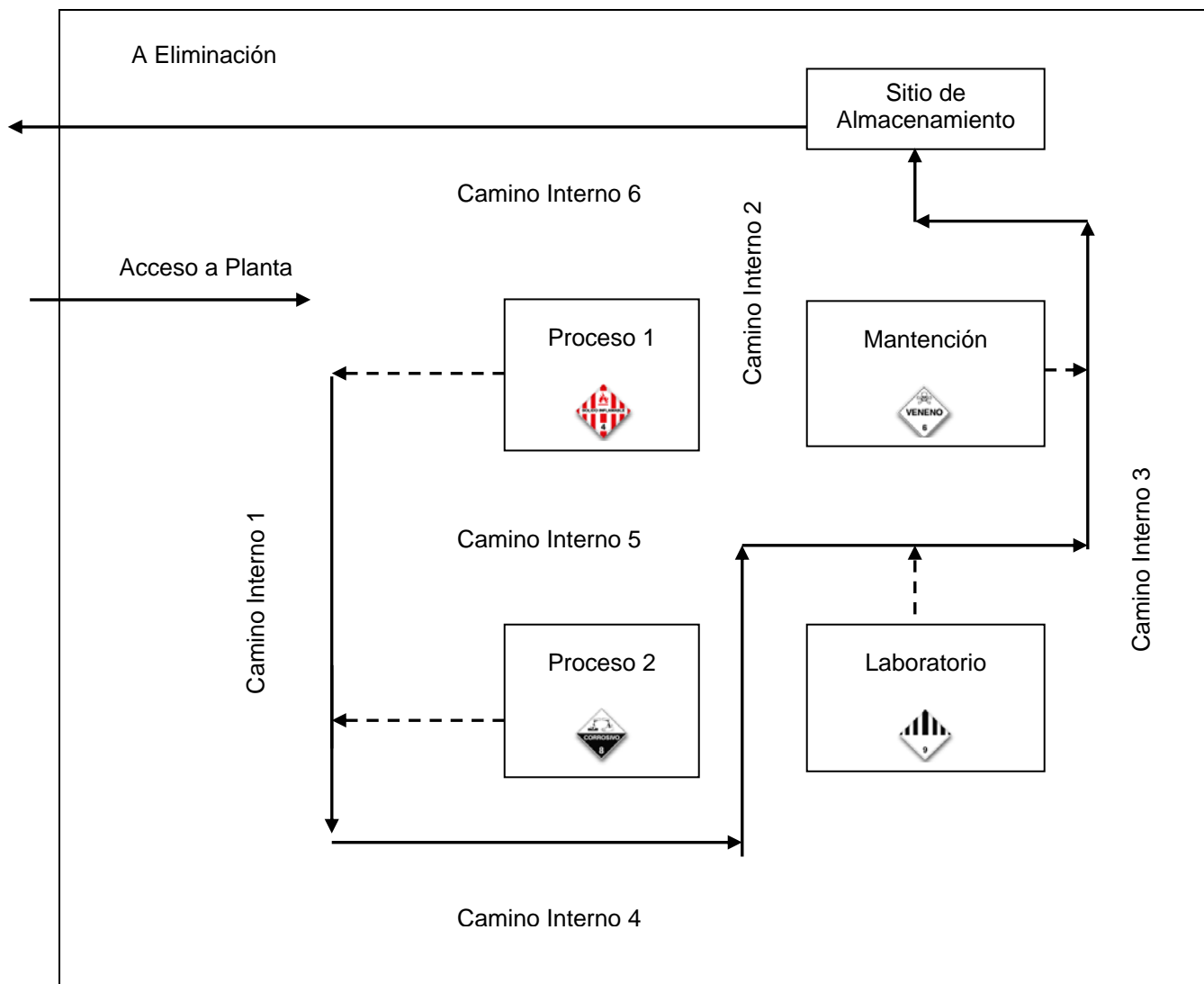
Figura N° 7: Plano de Ruteo de Recolección de Residuos Peligrosos
